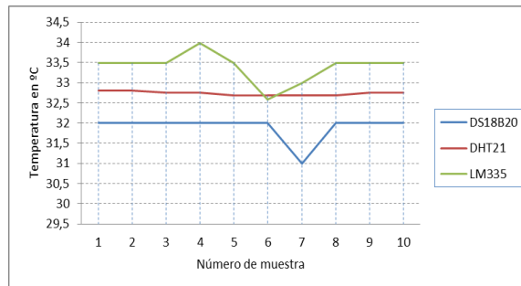
Fig. 5. Comparación sensores de temperatura DS18B20, DHT21, LM335
