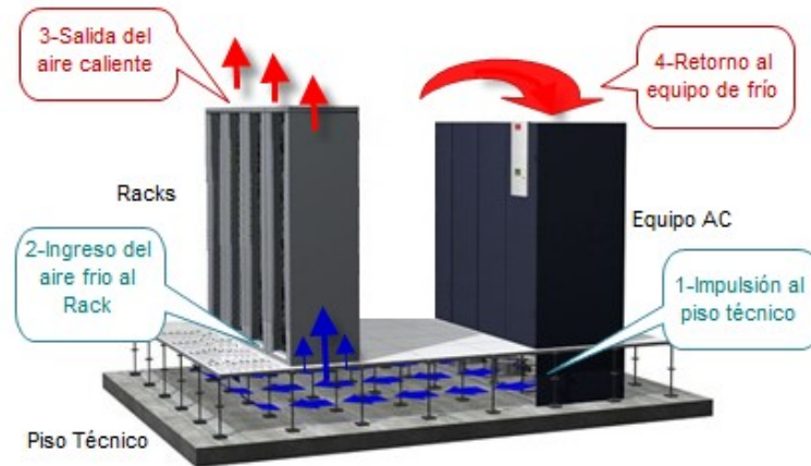
Fig. 4. Ciclo de acondicionamiento del aire
