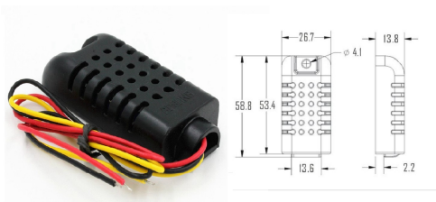
Fig. 6. Sensor de humedad y temperatura digital AM2301
