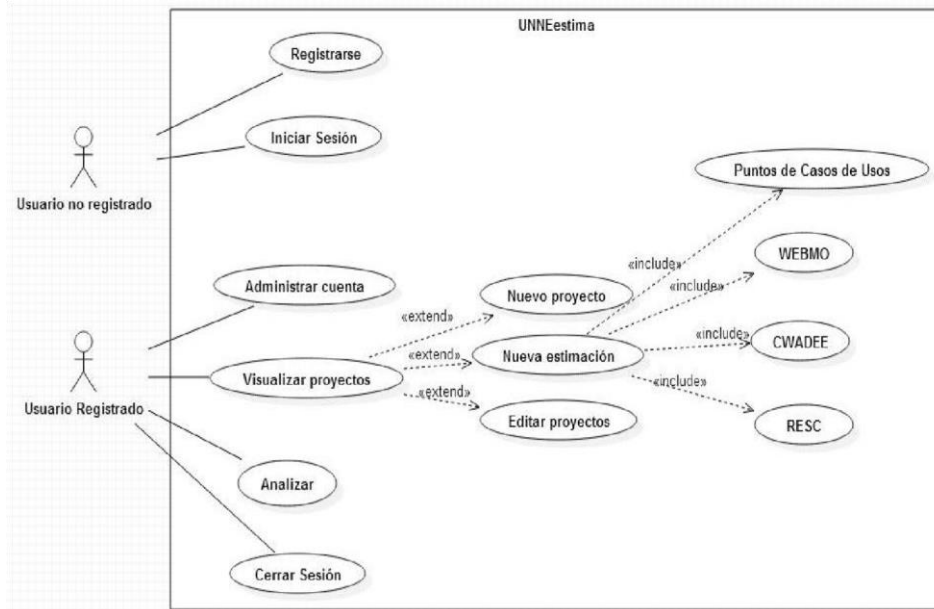
Fig. 1. Diagrama de casos de usos de la aplicación.
